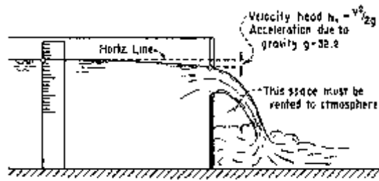
SECTION ON LONGITUDINAL CENTERLINE
